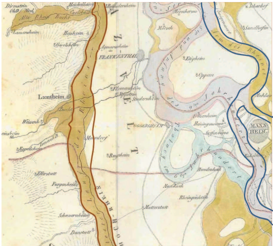
Abb. 1.2 (Karte 2): Ausschnitt aus einer Karte historischer Rheinverläufe von F. Mone von 1826 [11]; die braunen Uferlinien links sind Korrekturen des Autors; die blauen Linien rechts markieren den heutigen Rheinverlauf
